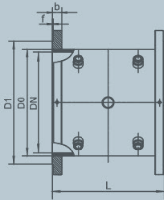
■ CRL-GC插入式超声热量表选配管段图尺寸表—四声路
