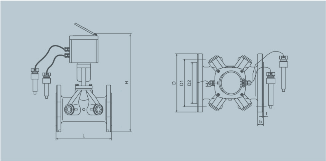
■ 法兰连接外形尺寸 (DN32~DN300)
