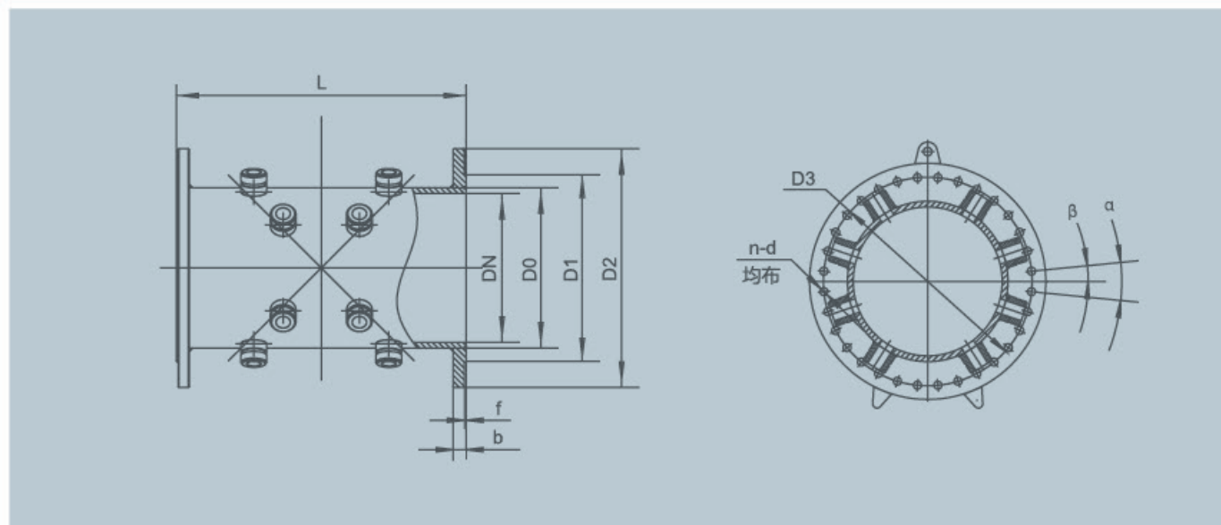
■ CRL-G插入式超声热量表(多声路)管段图尺寸表
