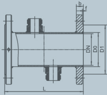
■ CRL-G插入式超声热量表选配管段图尺寸表—单声路
