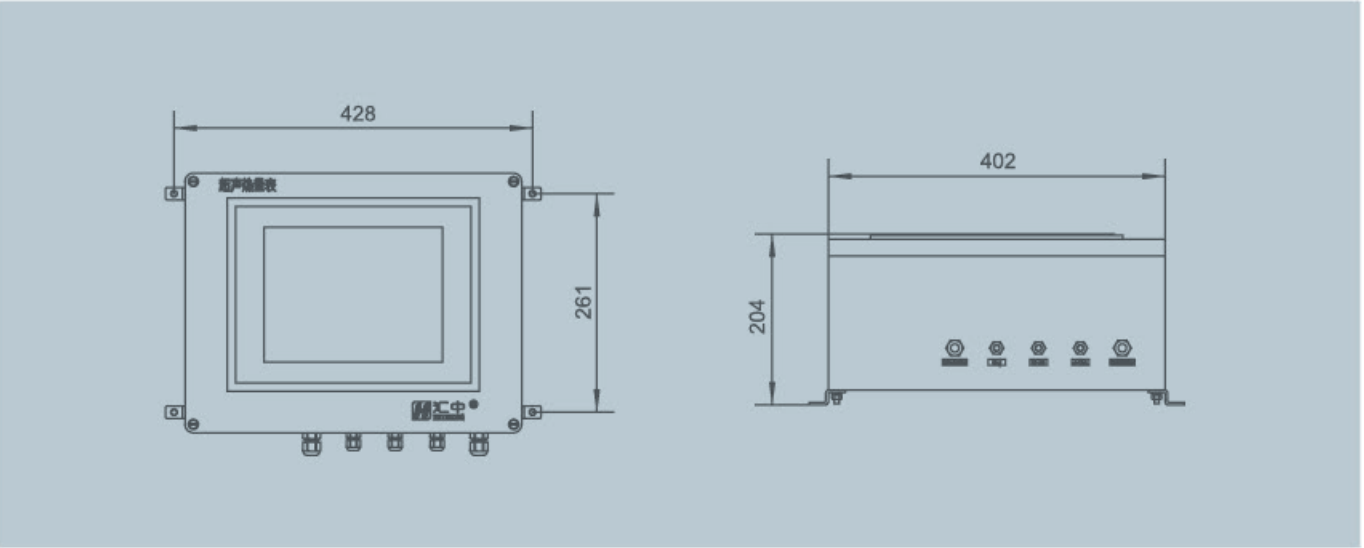
■ 多声路超声热量监测系统外形尺寸（mm）
