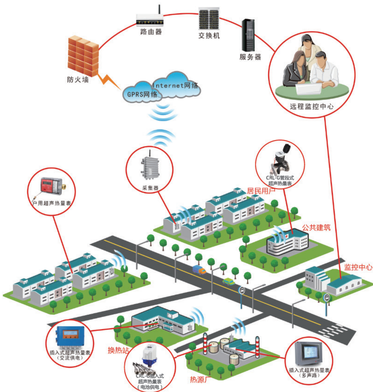
供热计量管理系统组网示意图
