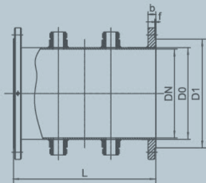
■ CRL-G插入式超声热量表选配管段图尺寸表—双声路
