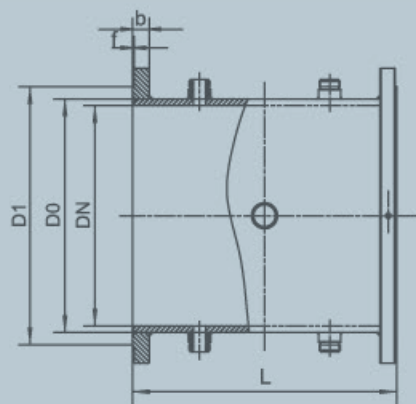
■ CRL-GC插入式超声热量表选配管段图尺寸表—双声路
